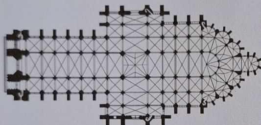
Cattedrale di Notre-Dame di Amiens, pianta.
