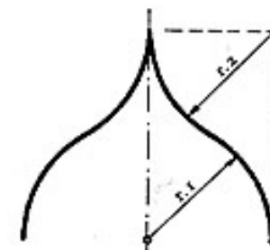
Arco inflesso o carenato, policentrico composto, III 9.
