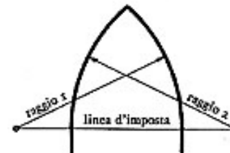
Arco a lancetta, acuto rialzato, III 7.
