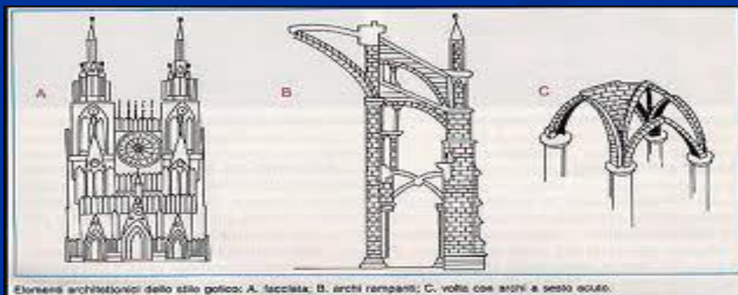
Esempi architettonici dello stile gotico: A. facciata; B. archi rampanti; C. volta con archi a sesto acuto.
