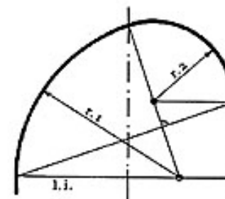
Arco rampante o a collo d'oca, III 15.
