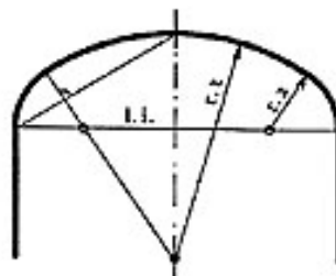
Arco ribassato policentrico («anse de panier»), III 4.
