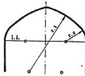
Arco «Tudor» policentrico ribassato, III 8.
