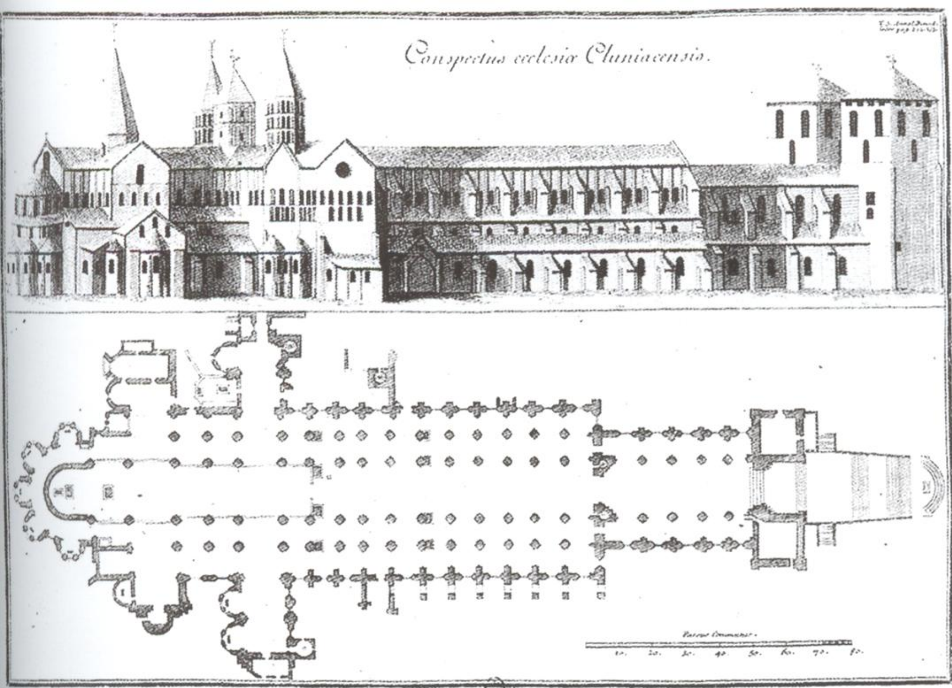
Pianta e sezione di Cluny III (da Mabillon, Annales ordinis benedicti , 1713)
