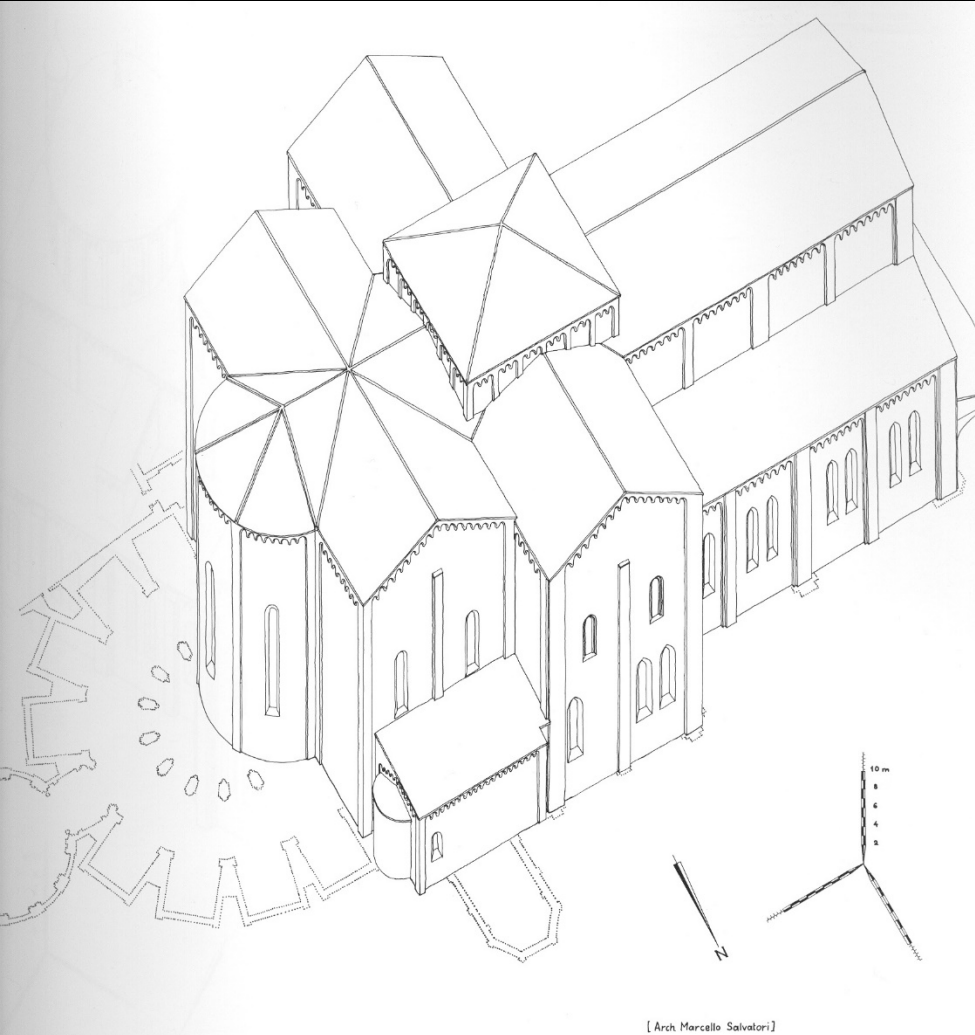
207. Ricostruzione assonometrica della Basilica nell'anno 1263. E' indicata anche la pianta della Basilica attuale.
