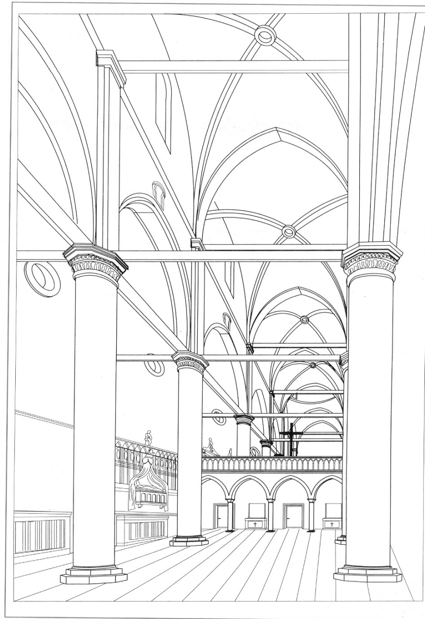
4. Venezia, chiesa dei Santi Giovanni e Paolo. Rappresentazione ipotetica dell'alzato e del tramezzo (disegno di E. Merlo). Nella ricostruzione sono visibili la porta centrale affiancata dai due altari e uno dei due passaggi laterali (navatella nord).
