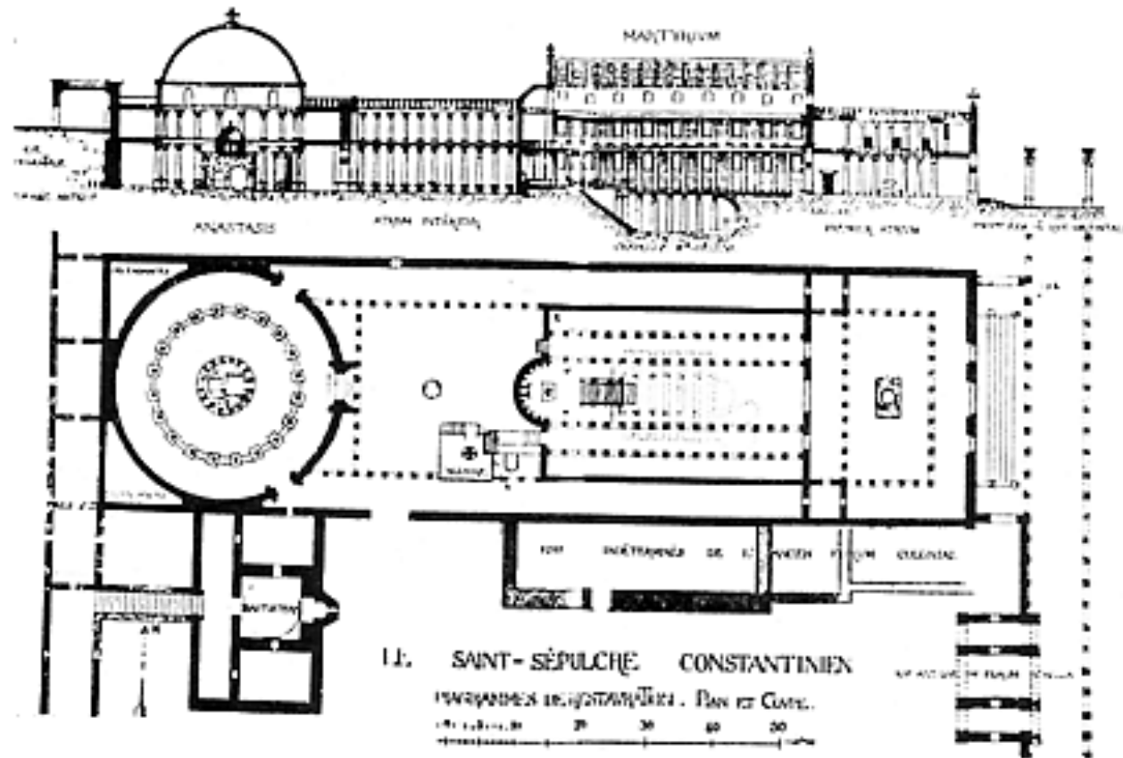
Pianta e sezione del S. Sepolcro di Gerusalemme.
